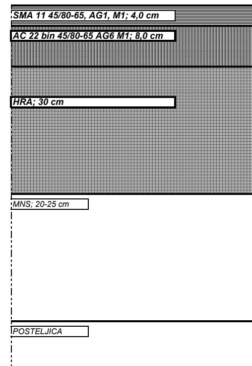
SANACIJA VOZNOG TRAKA, TIP B
