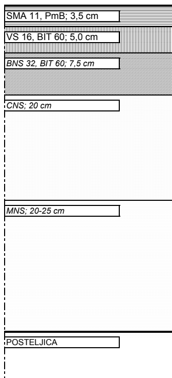
POSTOJEĆA KONSTRUKCIJA
