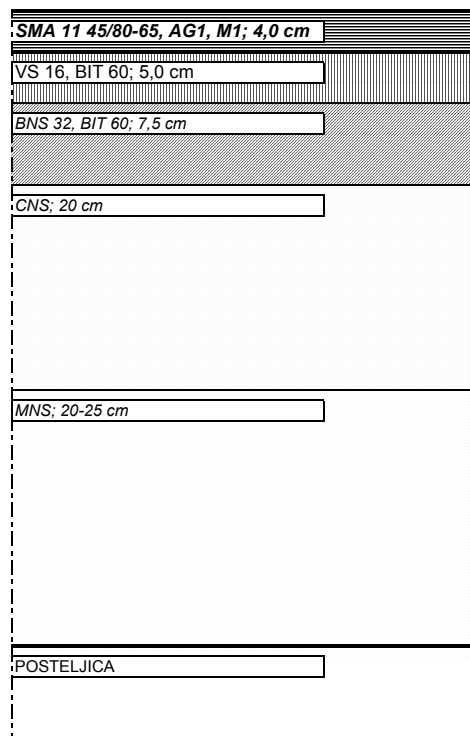
SANACIJA PRETJECAJNOG TRAKA
