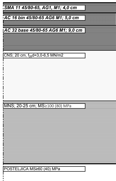
SANACIJA VOZNOG TRAKA, TIP A
